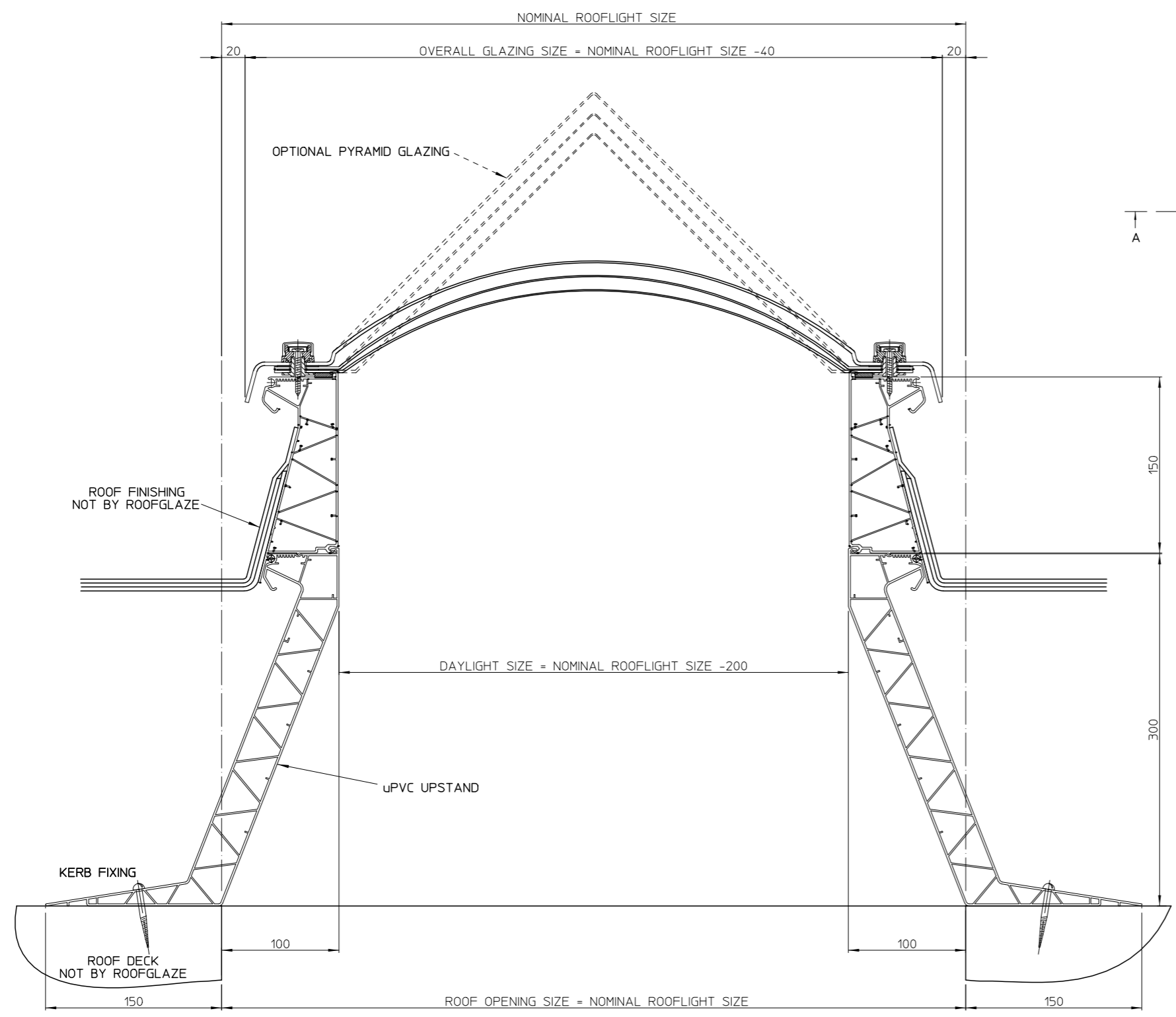
SECTION A-A
