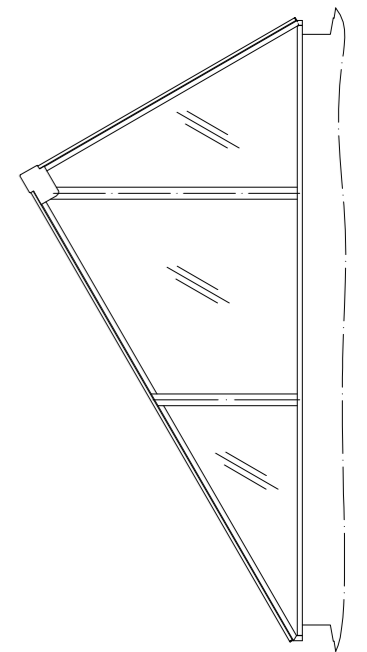
END ELEVATION
