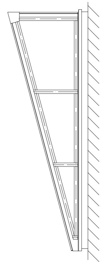
END ELEVATION
