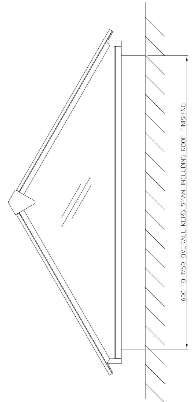
END ELEVATION
