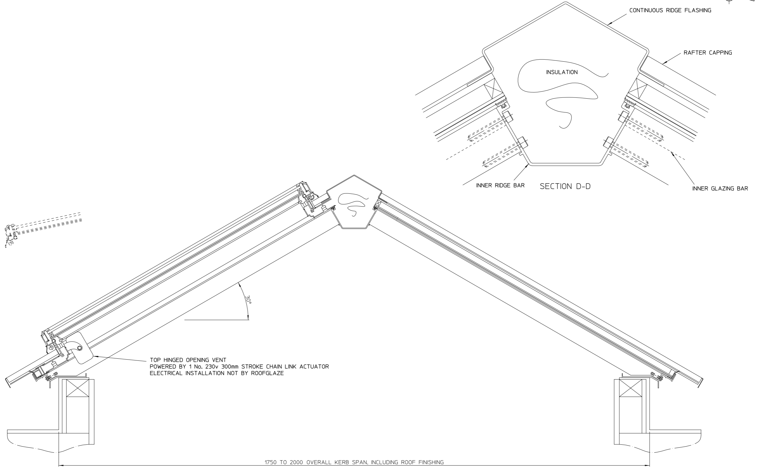
SECTION A-A
