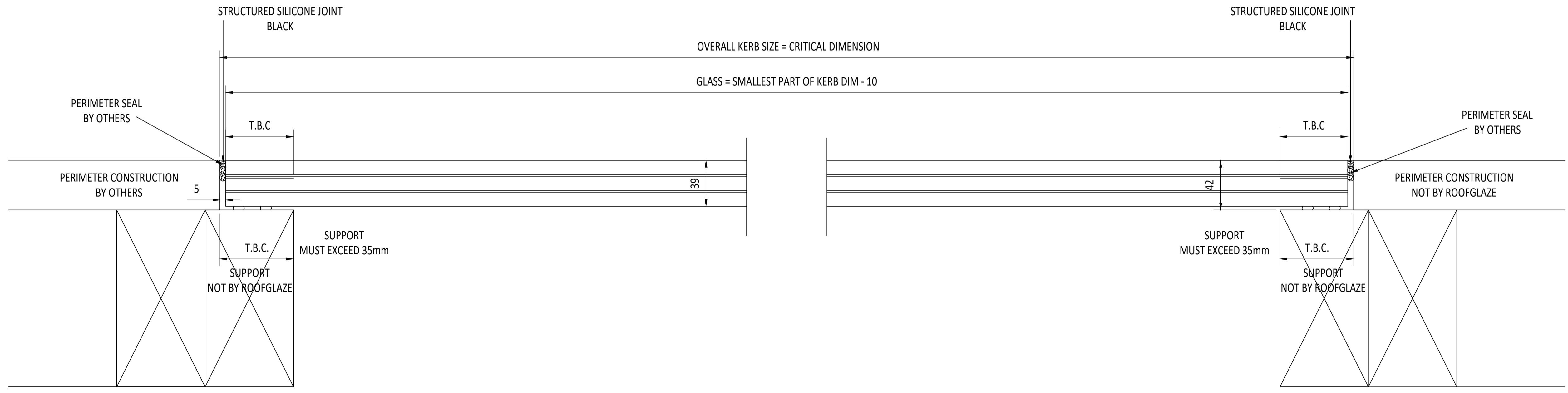
SECTION A-A
