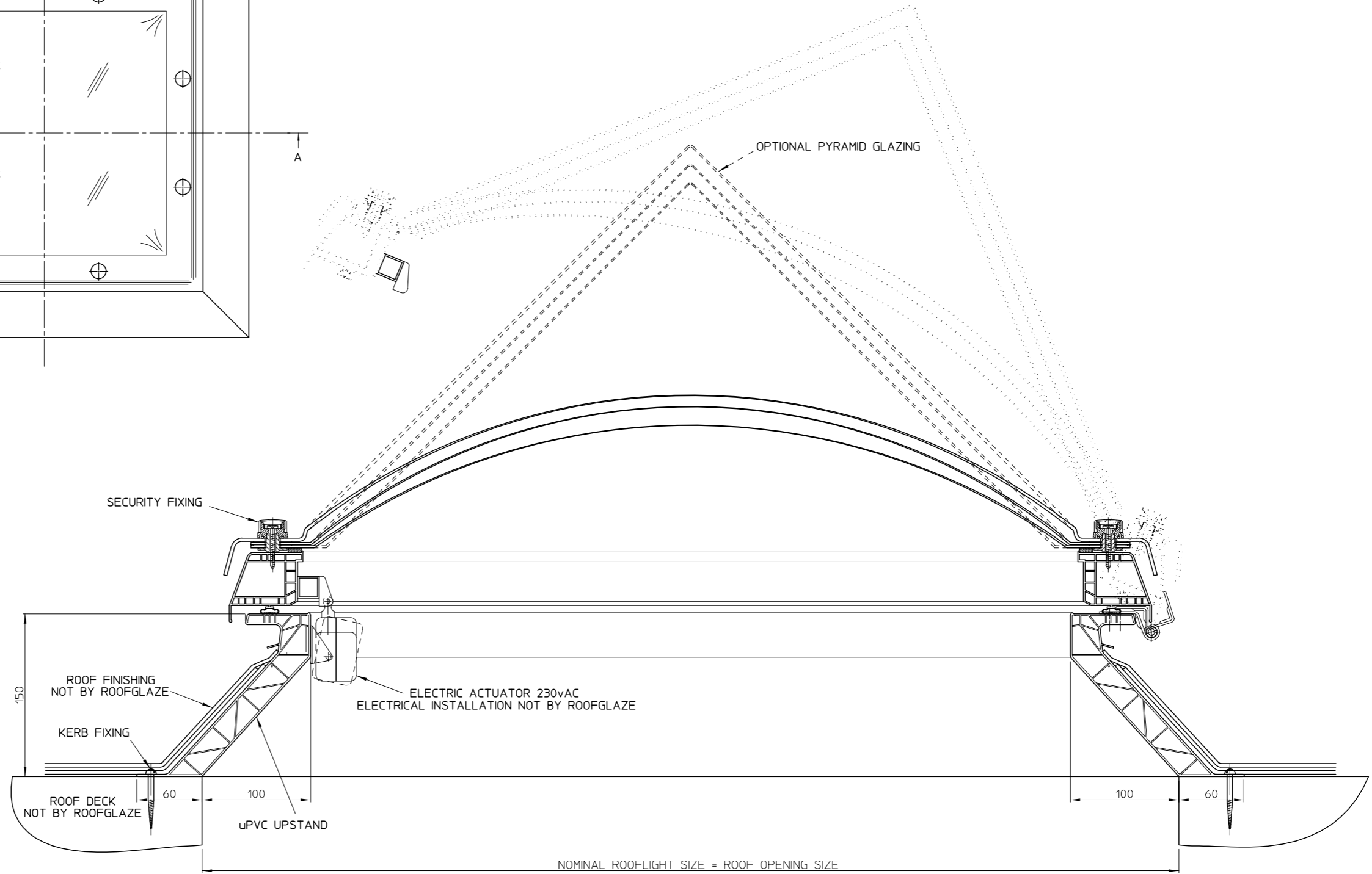
SECTION A-A
