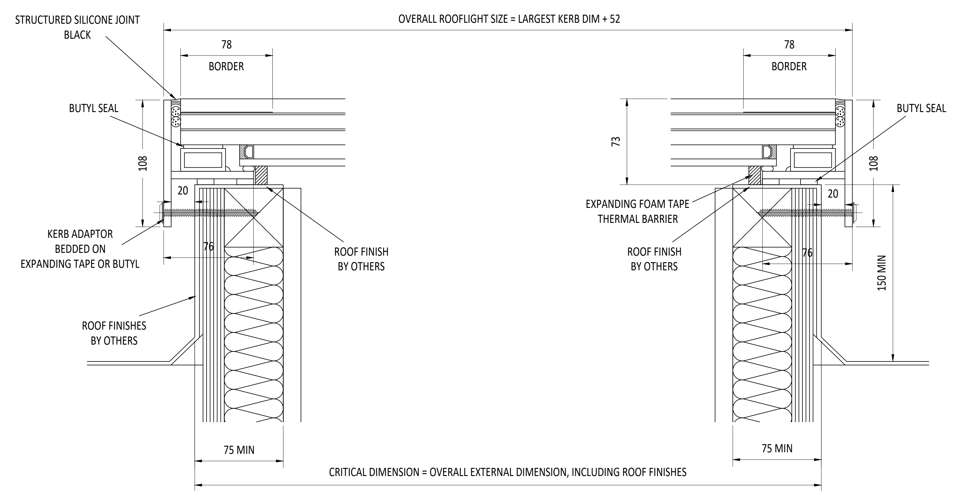
SECTION A-A
